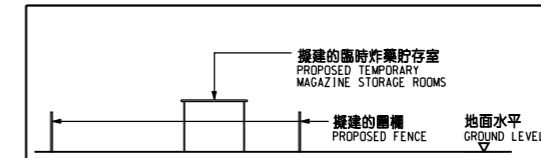
切面圖 SECTION B-J 不設比例 NOT TO SCALE
