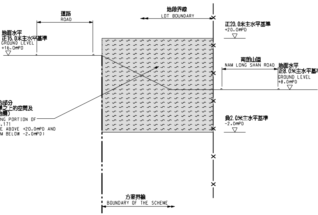
切面圖 SECTION AV 不按比例 NOT TO SCALE
