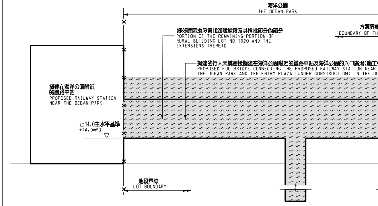
切面圖 SECTION AT 不依比例 NOT TO SCALE
