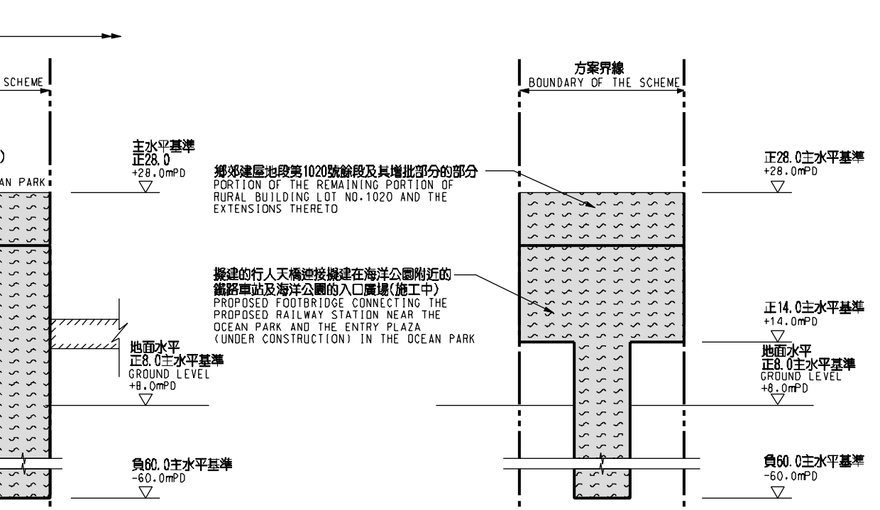
切面圖 SECTION AU 不依比例 NOT TO SCALE
