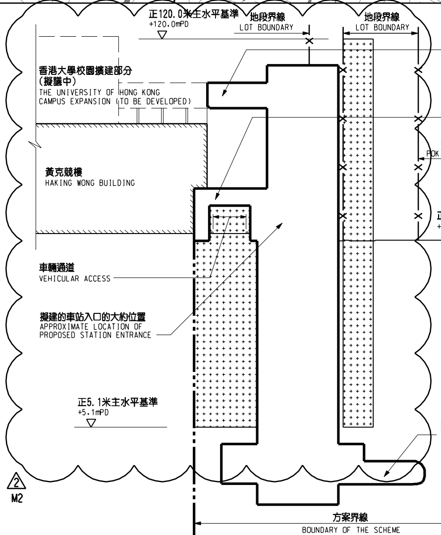
切面圖 SECTION B 不按比例 NOT TO SCALE
